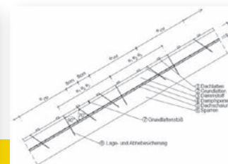
Systemskizze 80 mm – 120 mm
